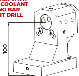
137-00300 - (Ø40 mm)
