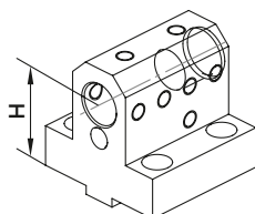
W1417 D25 - H=55 mm (Ø25 mm) W4437 D25 - H=75 mm (Ø25 mm)
