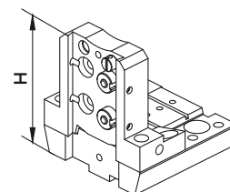
121-22076 (h=32 mm - H=100 mm)
